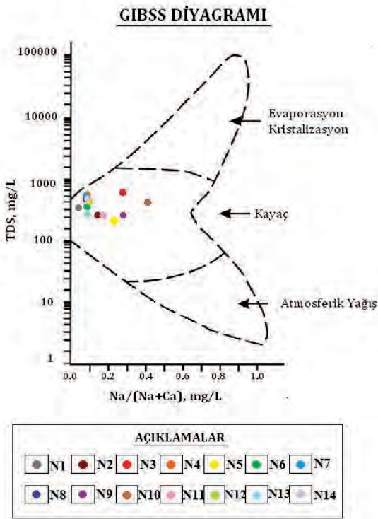
Şekil 7. Gibbs diyagramı.
